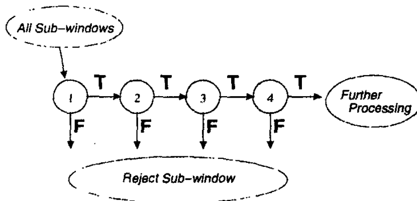
Gambar 1 Skema deteksi cascade
